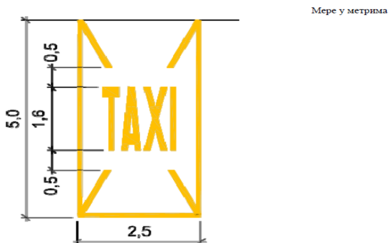
Слика 6: Начин обележавања паркинг места за паркирање појединачног такси возила у случају подужног паркирања (под углом од 0^\circ ) – СРПС У.С4.233_2020.
