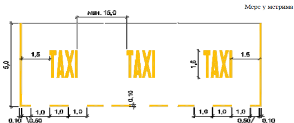
Слика 3: Начин обележавања више паркинг места за такси возила у случају управног паркирања (под углом од 90^\circ ) – СРПС У.С4.233_2020.
