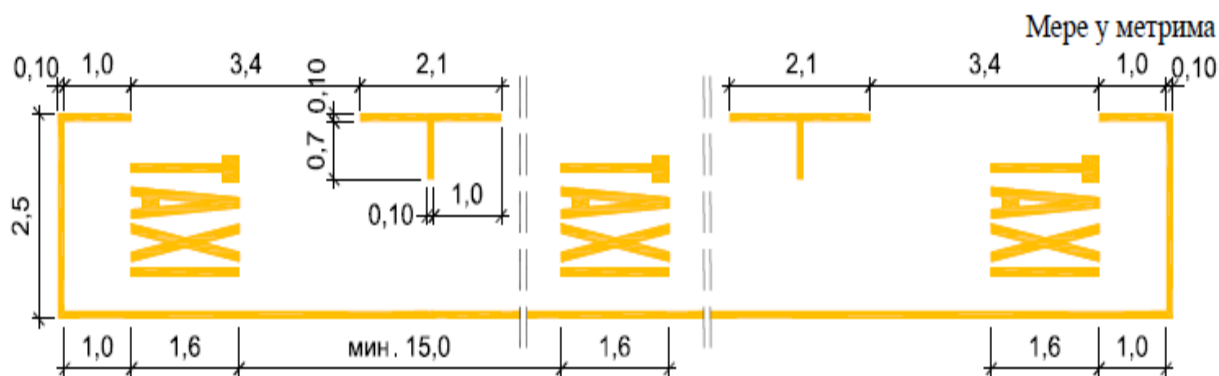
Слика 5: Начин обележавања више појединачних паркинг места за такси возила у случају управног паркирања (под углом од 90^\circ ) – СРПС У.С4.233_2020.
