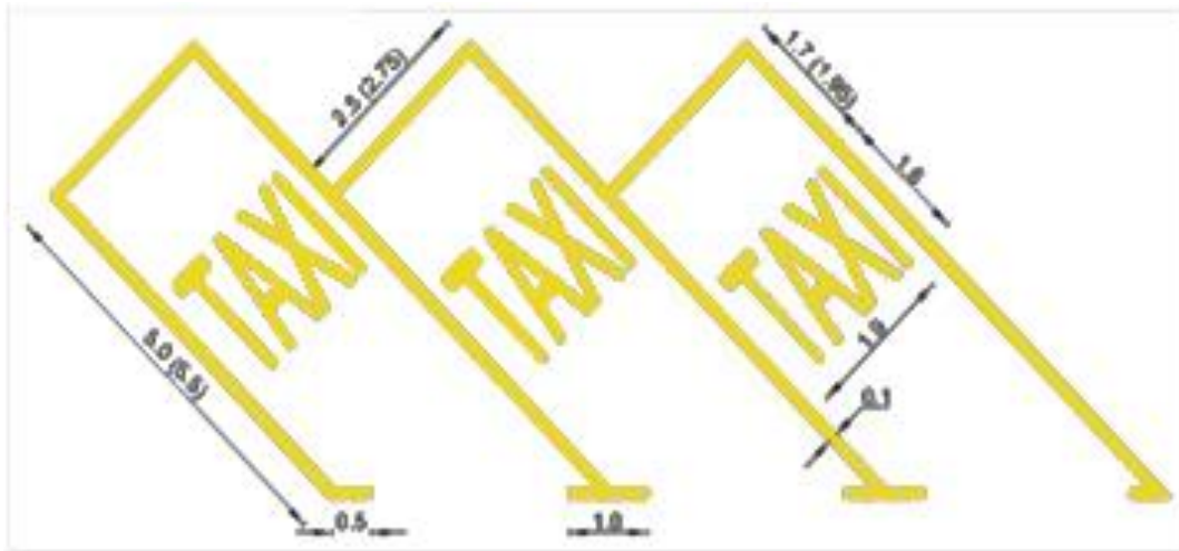
Слика 8: Начин обележавања паркинг места за такси возила у случају косог паркирања (под углом мањим од 90^\circ )
