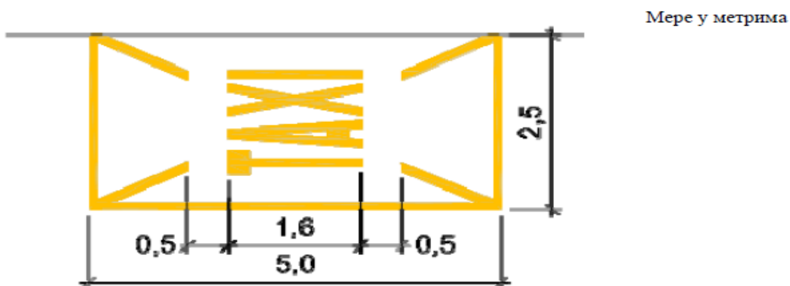
Слика 7: Начин обележавања паркинг места за паркирање појединачног такси возила у случају управног паркирања (под углом од 90^\circ ) – СРПС У.С4.233_2020.
