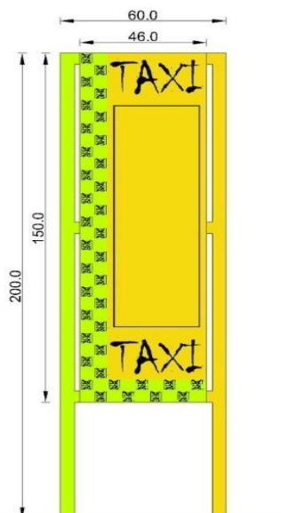
Слика 9: Скица наменске огласне табле
