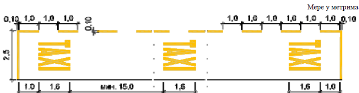
Слика 2: Начин обележавања више паркинг места за такси возила у случају подужног паркирања (под углом од 0^\circ ) – СРПС У.С4.233_2020.
