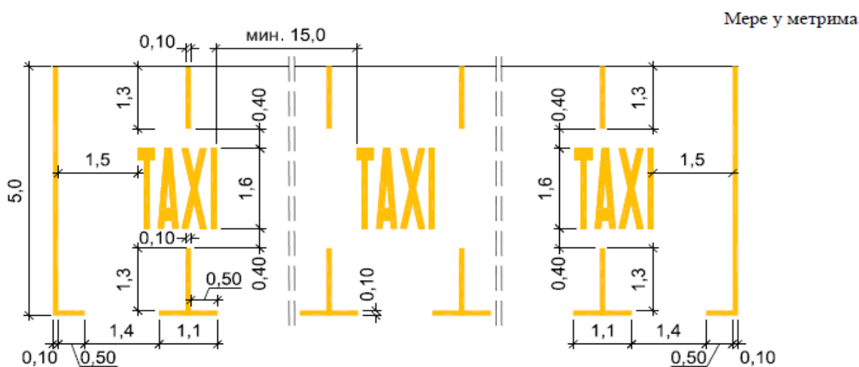
Слика 4: Начин обележавања више појединачних паркинг места за такси возила у случају подужног паркирања (под углом од 0^\circ ) – СРПС У.С4.233_2020.
