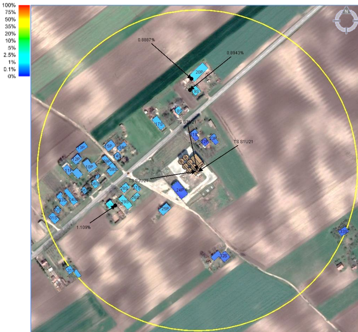
Slika 6.13. Izloženost od radio-sistema UMTS2100 I LTE800 BS „SUU114, SUO114 MIŠIĆEVO“ operatera „Telekom Srbija“ na nivoima najizloženijih spratova
