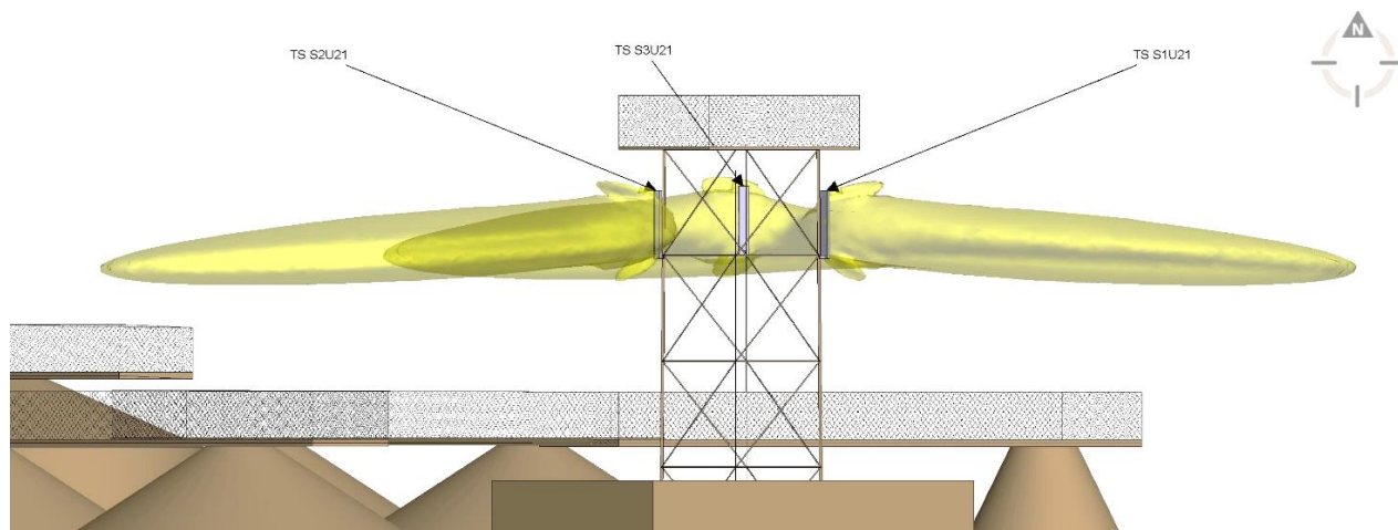
Slika 6.2. Kontrolisana zona, horizontalan pogled na antenu sa južne strane
