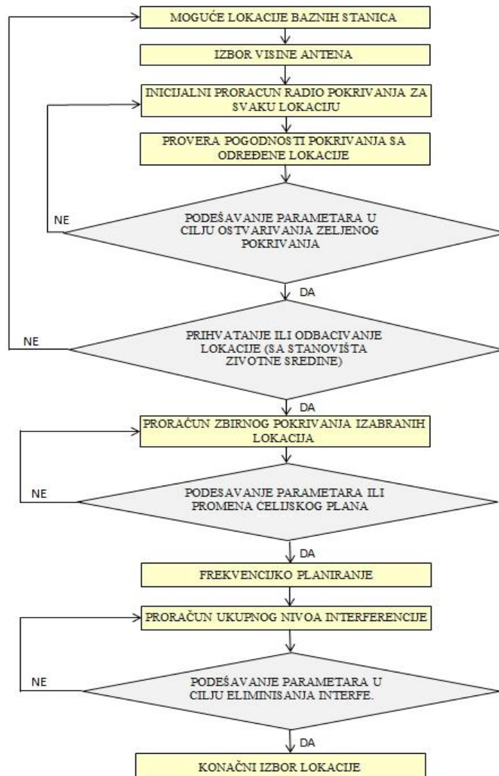
Slika 4.1 Procedura izbora mikrolokacija baznih stanica
