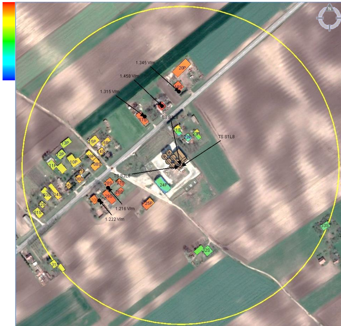
Slika 6.12. Jačina električnog polja radio-sistema LTE800 bazne stanice „SUU114, SUO114 MIŠIĆEVO” operatora „Telekom Srbija“ na nivoima najizloženijih spratova
