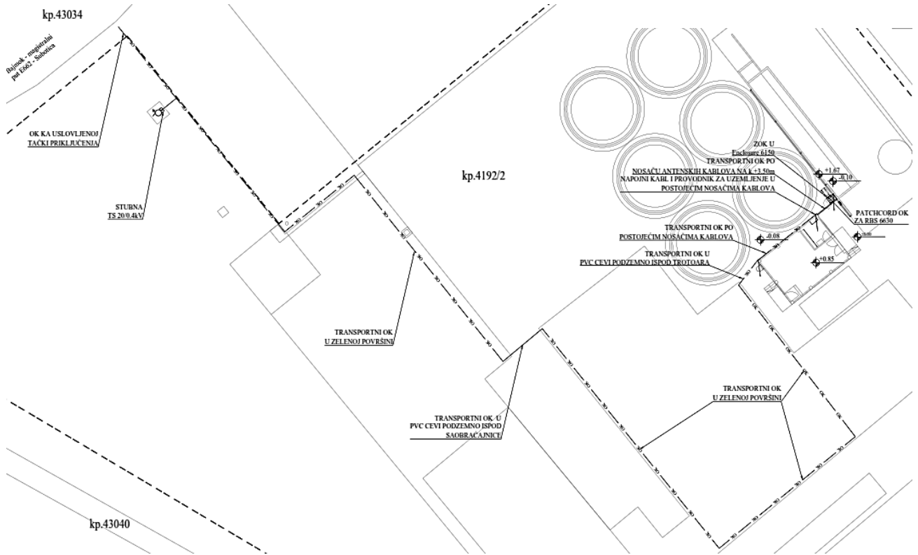
Slika 4.3 Trasa kablova za prenos
