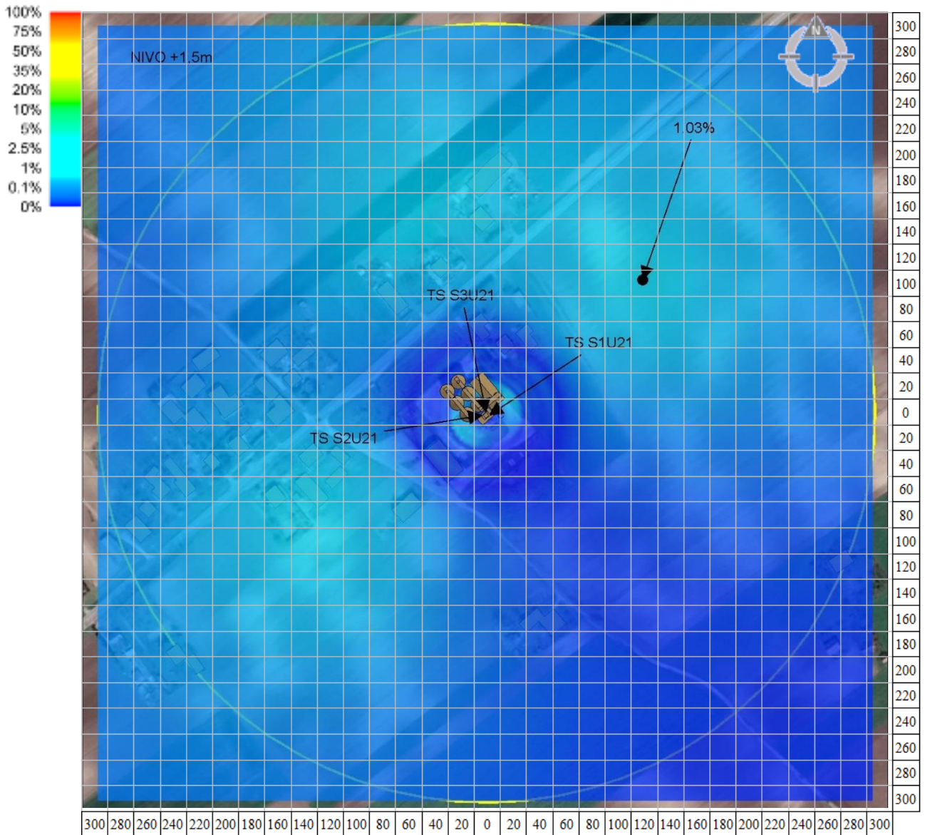
Slika 6.10. Jačina električnog polja radio-sistema UMTS2100 i LTE800 bazne stanice „SUU114, SUO114 MIŠIĆEVO” operatora „Telekom Srbija“ na nivou 1,5 m
