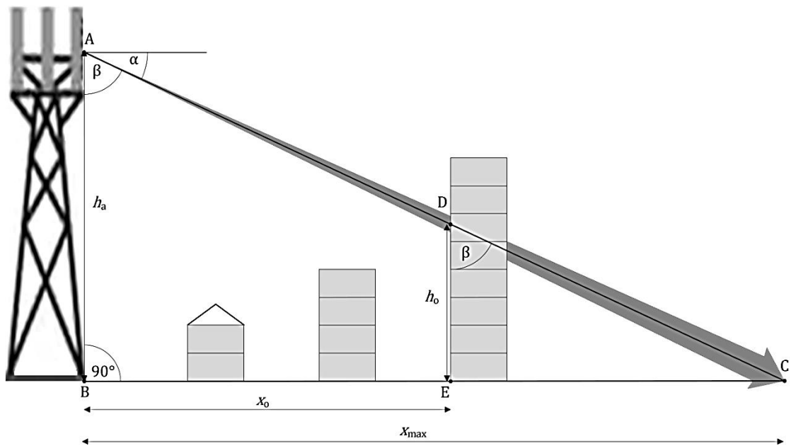
Slika 6.2C Određivanje najizloženijeg sprata objekta u zoni povećane osetljivosti
