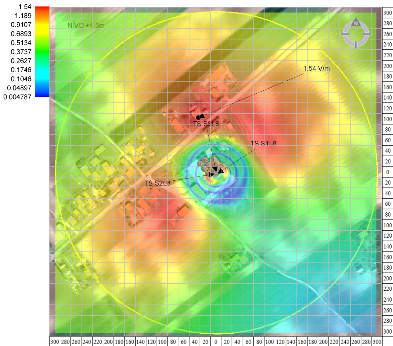
Slika 6.9. Jačina električnog polja radio-sistema LTE800 bazne stanice „SUU114, SUO114 MIŠIĆEVO” operatora „Telekom Srbija” na nivou 1,5 m
