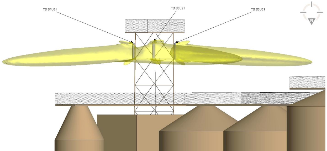
Slika 6.3. Kontrolisana zona, horizontalan pogled na antenu sa severne strane
