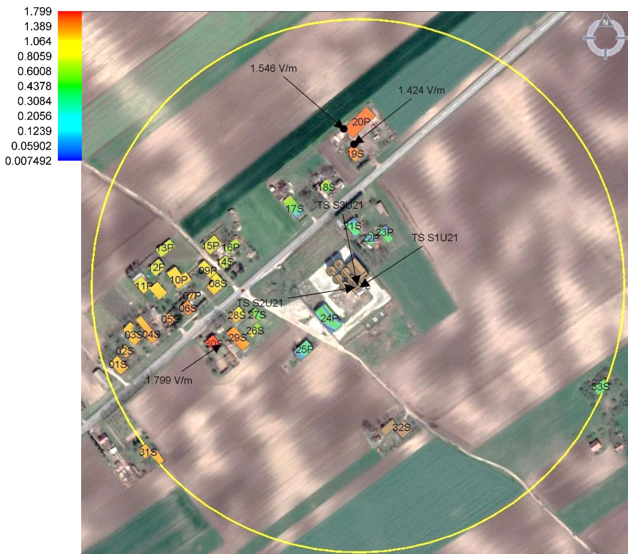
Slika 6.11. Jačina električnog polja radio-sistema UMTS2100 bazne stanice „SUU114, SUO114 MIŠIĆEVO” operatora „Telekom Srbija“ na nivoima najizloženijih spratova
