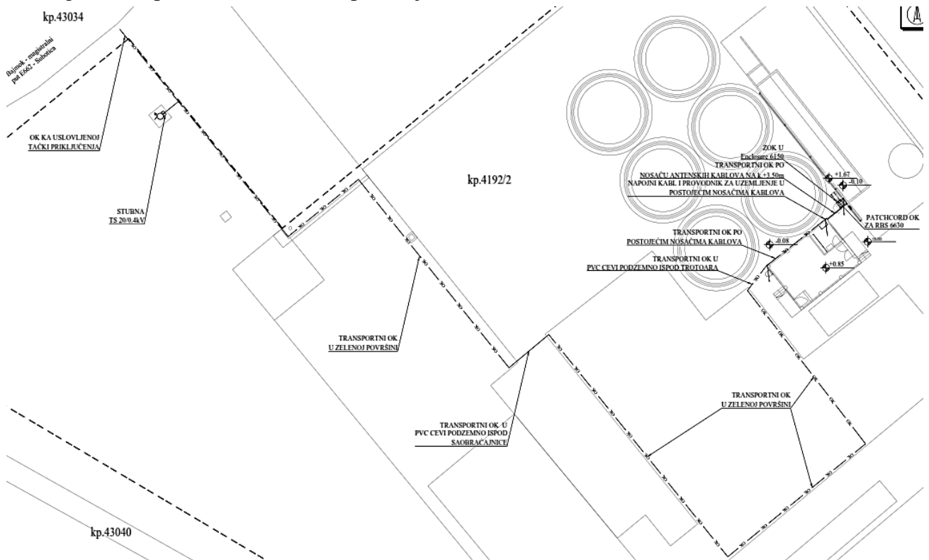
Slika 6.1. Šira situacija – trasa kablova za prenos
