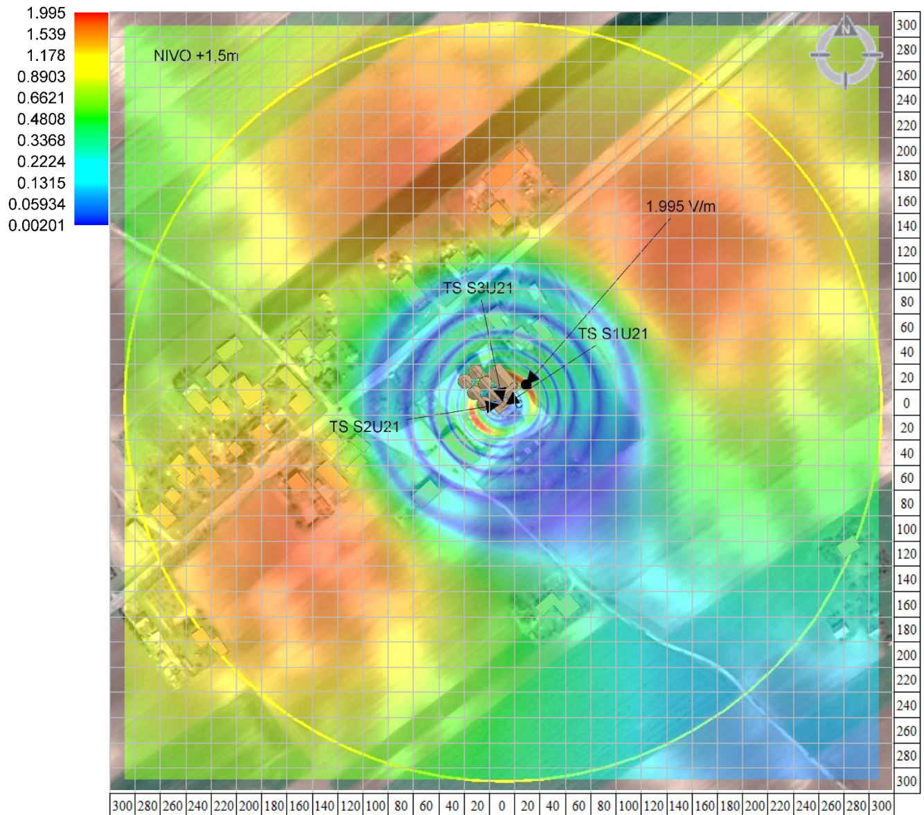
Slika 6.8. Jačina električnog polja radio-sistema UMTS2100 buduće bazne stanice “SUU114, SUO114 MIŠIĆEVO” operatora “Telekom Srbija” na nivou 1,5 m
